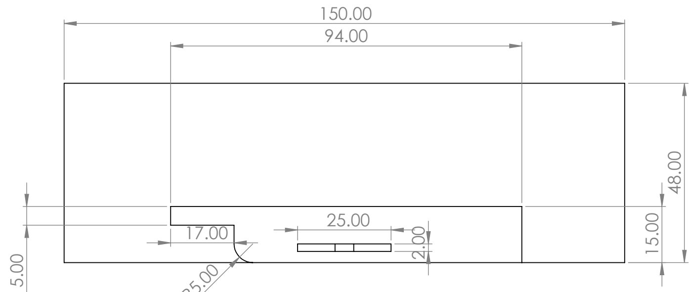
Vista Superior
